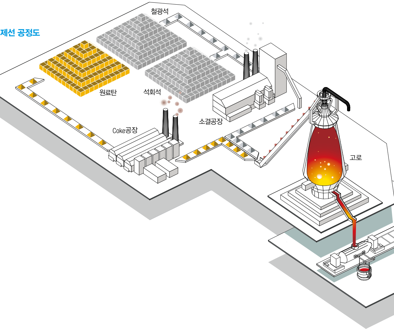
제선 공정별 상세 설명
