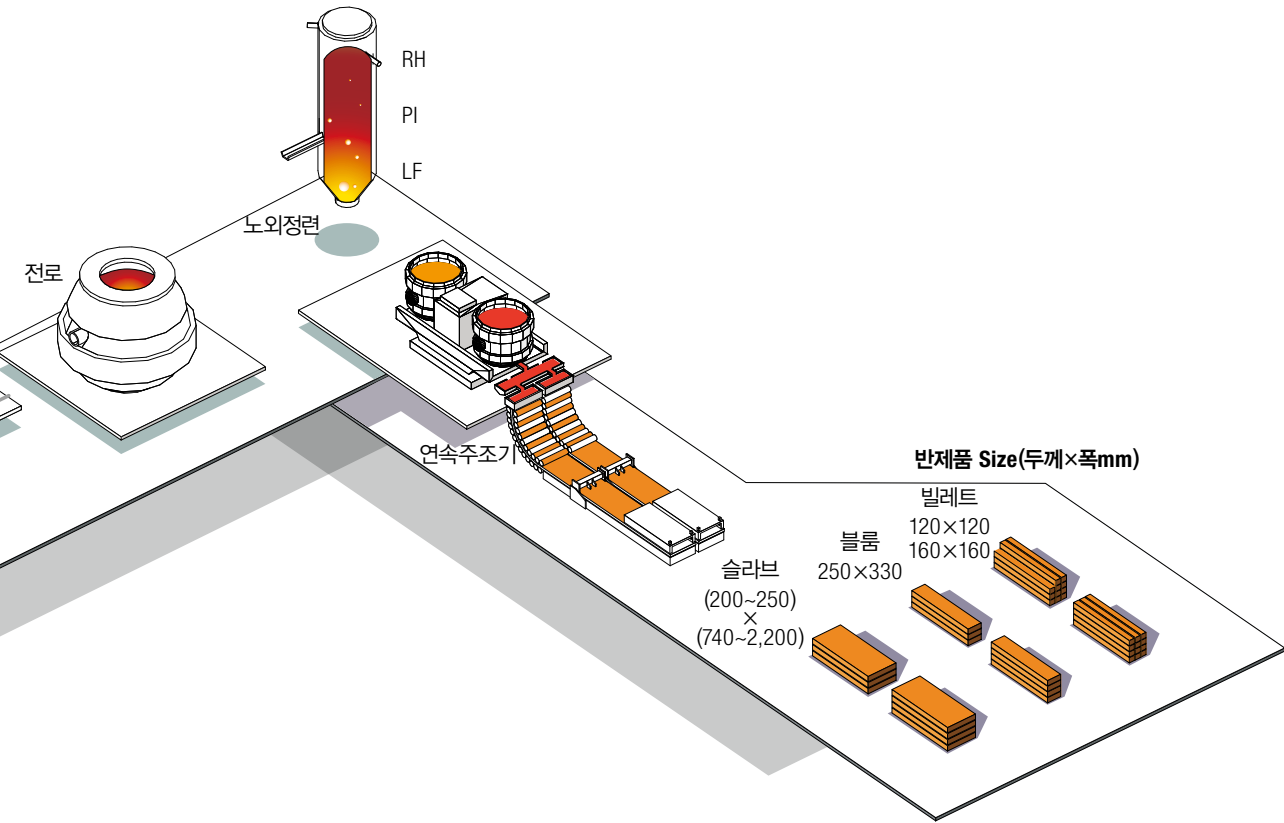
제강 / 연주 공정별 상세 설명
